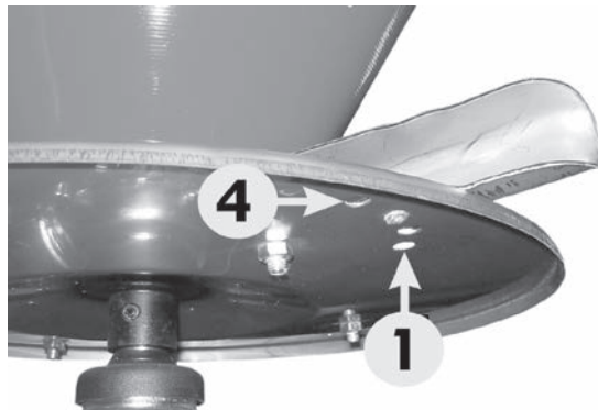
Ajuste paletas disco de distribución
